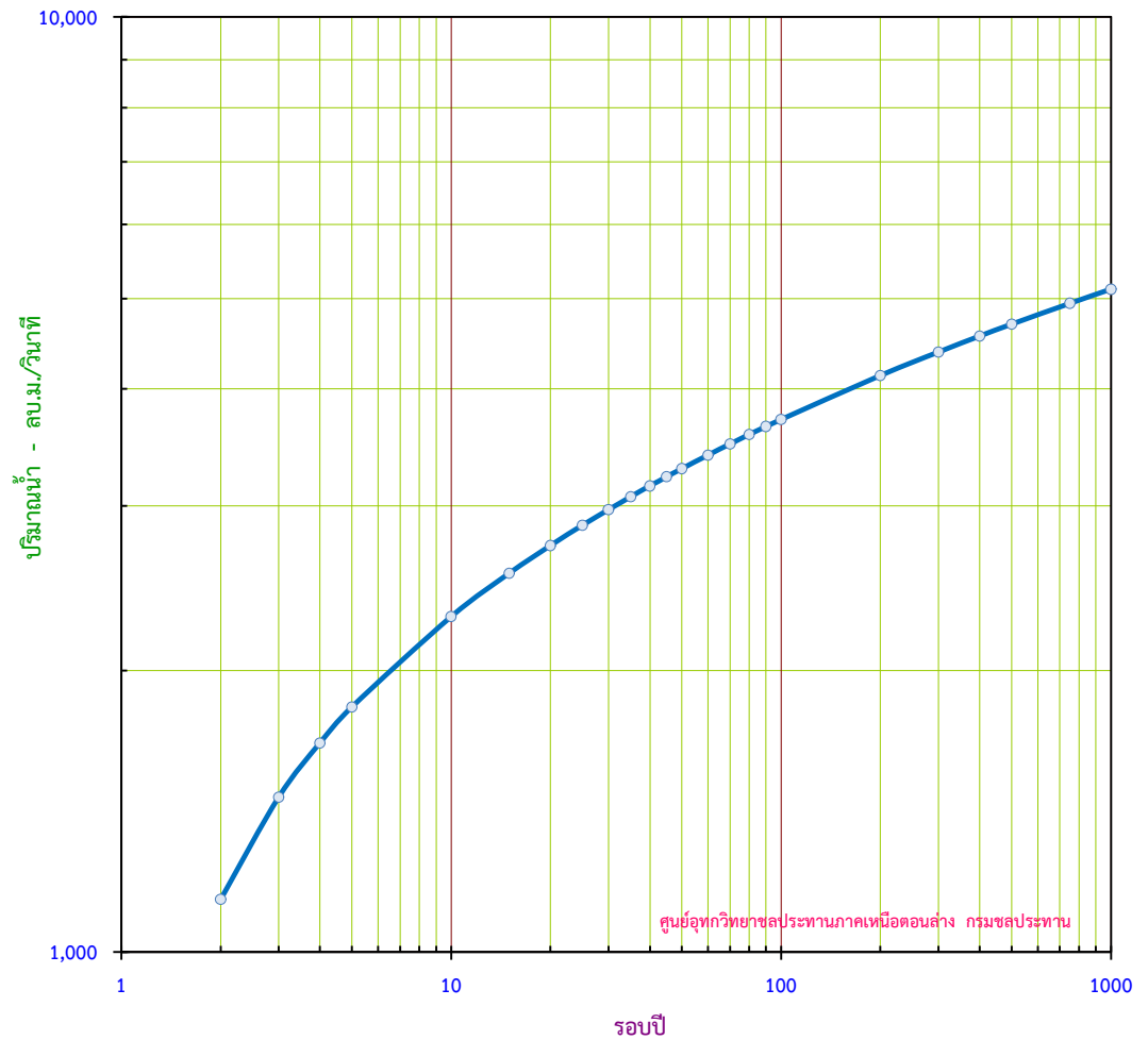
กราฟแสดง ปริมาณน้ำสูงสุดรายปี ขนาดรอบปีต่างๆ สถานี P.16 อ.ขามเฒ่า จ.กำแพงเพชร
